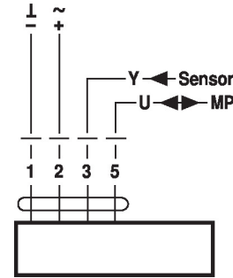
Külső kapcsolóérintkező csatlakozása
