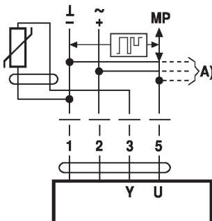
Passzív érzékelők csatlakozása
