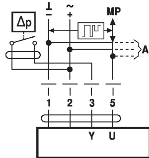
Külső kapcsolóérintkező csatlakozása
