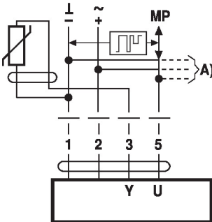
Passzív érzékelők csatlakozása
