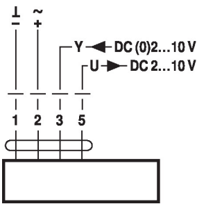
Aktív érzékelők csatlakoztatása
