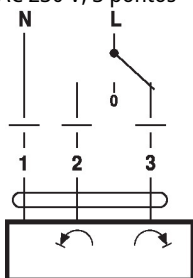
Kapcsolási rajz AC 230 V, 3 pontos
