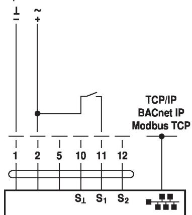
Kapcsolóérintkező csatlakozása
