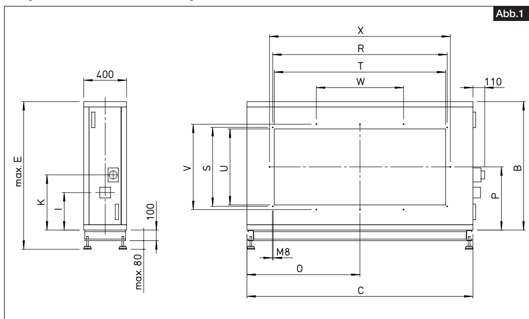
Abmessungen externe elektrische Nachheizung
