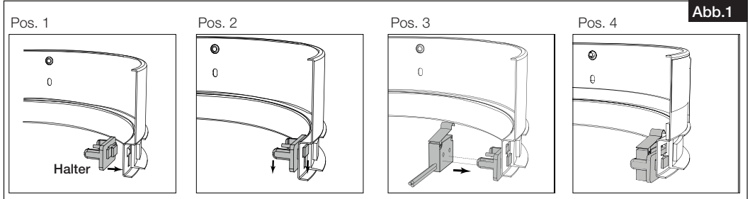
Abb. 2 Schmelzlot ersetzen
